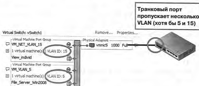
Рис. 2.24. Схема Virtual switch tagging
