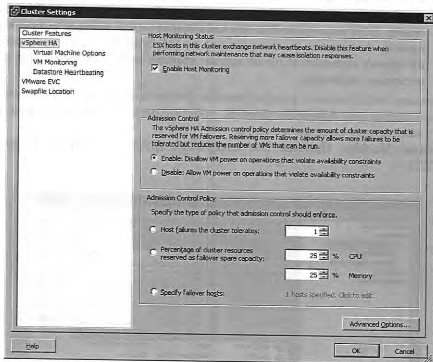
Рис. 7.1. Основные настройки кластера HA
