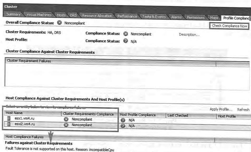
Рис. 7.17. Встроенная проверка кластера на соответствие требованиям FT
