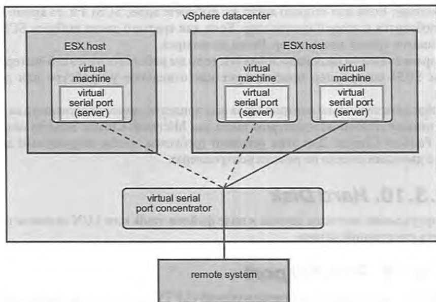
Рис. 5.13. Схема работы с концентратором последовательных портов Источник: VMware
