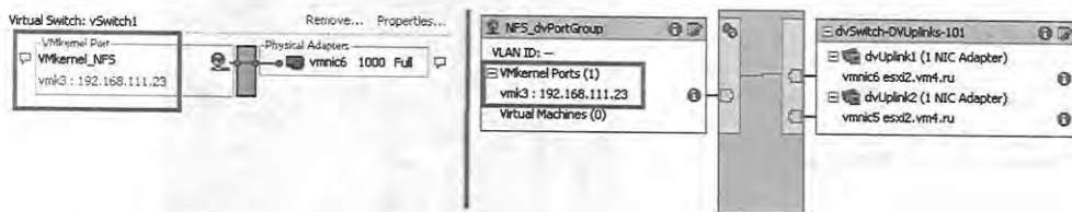
Рис. 3.2. Интерфейс VMkernel на стандартном или распределенном виртуальном коммутаторе
