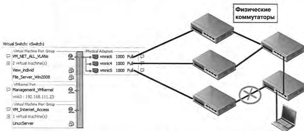
Рис. 2.33. Пример конфигурации сети, при которой имеет смысл использовать Beacon Probing
