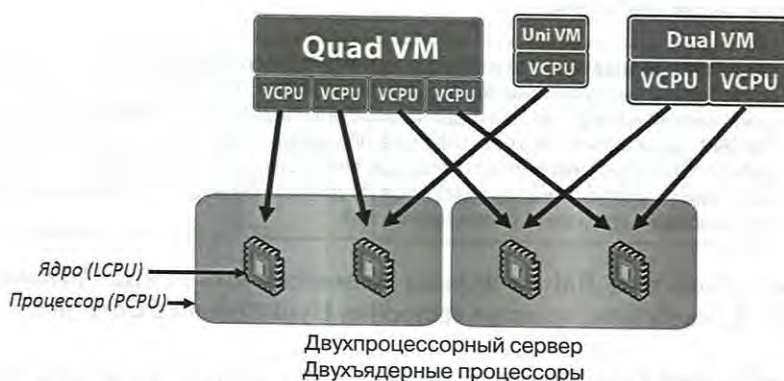
Рис. 6.23. Иллюстрация работы с процессорной подсистемой Источник: VMware
