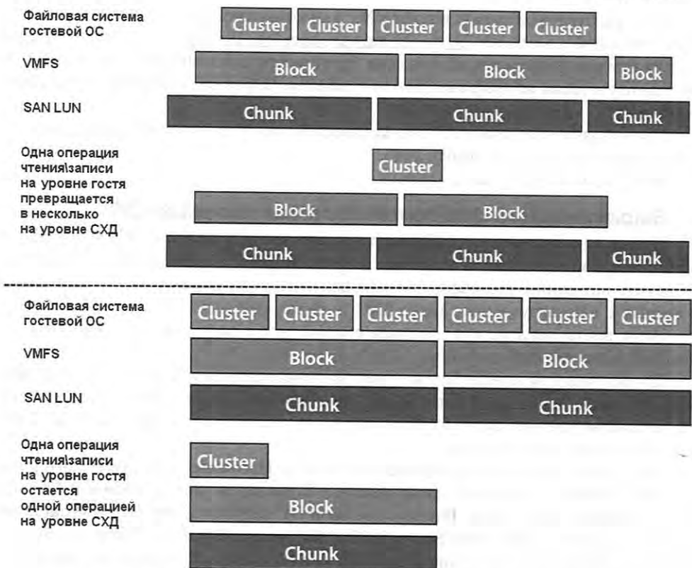
Рис. 5. 23. Иллюстрация выровненных и невыровненных разделов Источник: VMware
