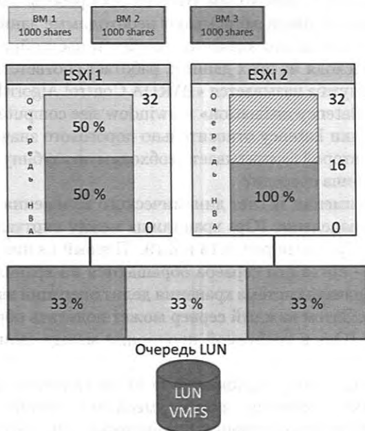
Рис. 6.19. Распределение операций ввода-вывода между VM разных серверов при включенном SIOC
