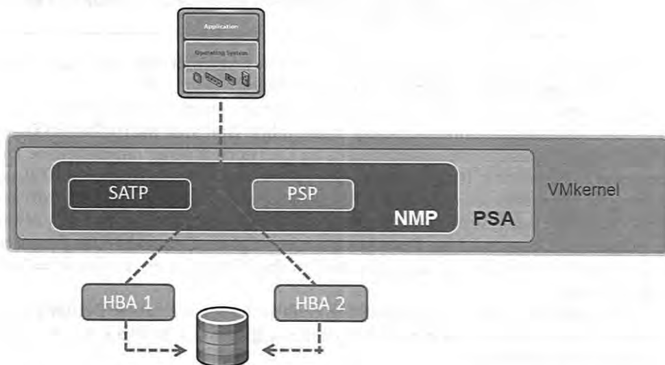
Рис. 3.10. Схема связей модулей гипервизора для работы с дисковой подсистемой Источник: VMware
