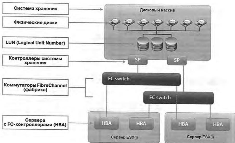
Рис. 3.6. Схема FC SAN Источник: VMware
