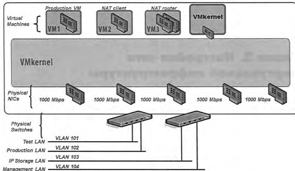
Рис. 2.1. Основные объекты сети «внутри» ESXi
