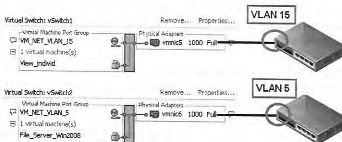
Рис. 2.23. Схема External switch tagging
