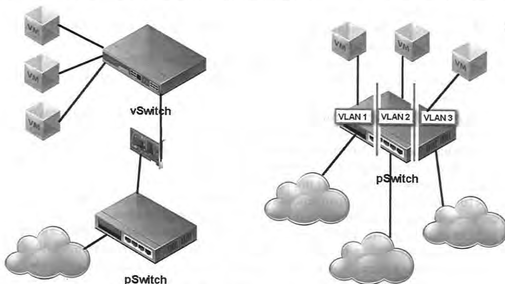
Рис. 2.22. Сервера (ВМ) подключены к одному коммутатору, но к разным VLAN
