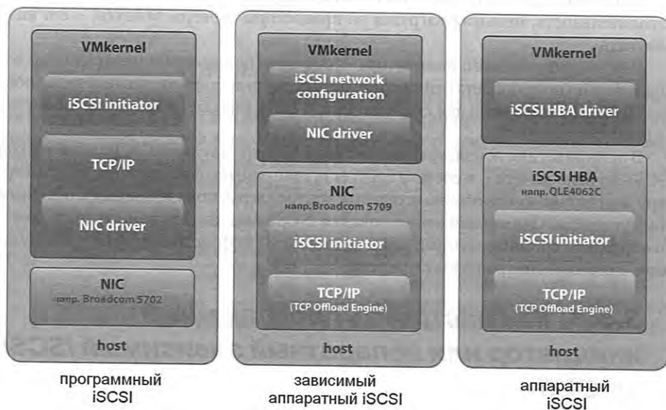
Рис. 3.15. Иллюстрация разницы между вариантами инициатора iSCSI Источник: VMware
