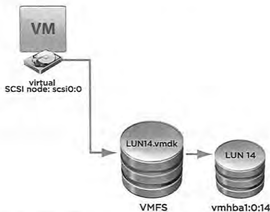
Рис. 3.29. Иллюстрация подключения RDM Источник: VMware
