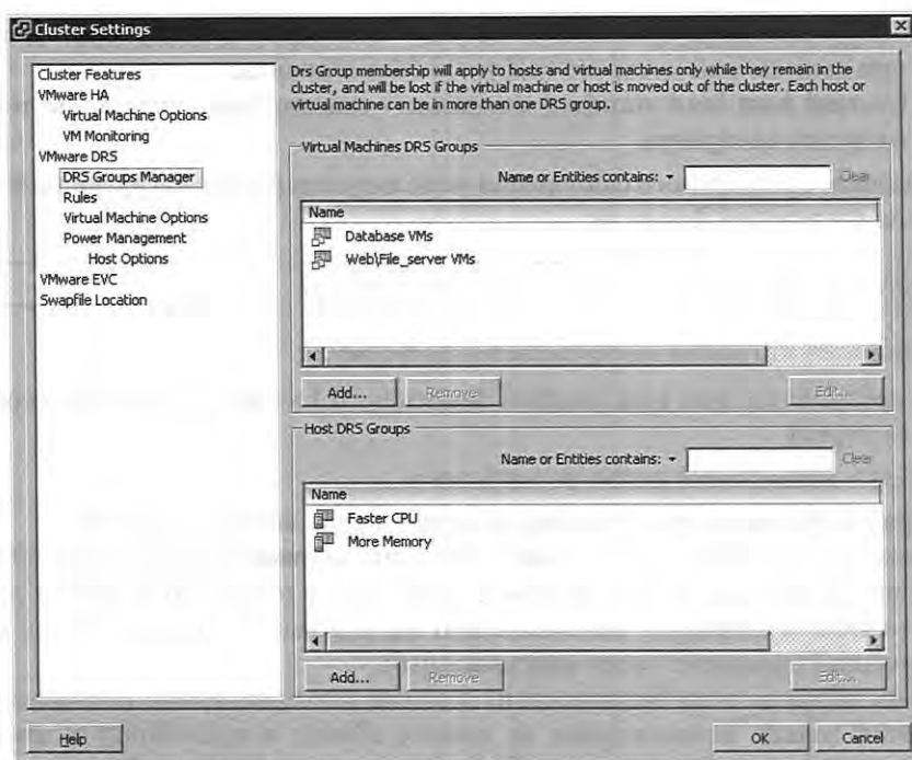
Рис. 6.62. Группы серверов и виртуальных машин для кластера DRS
