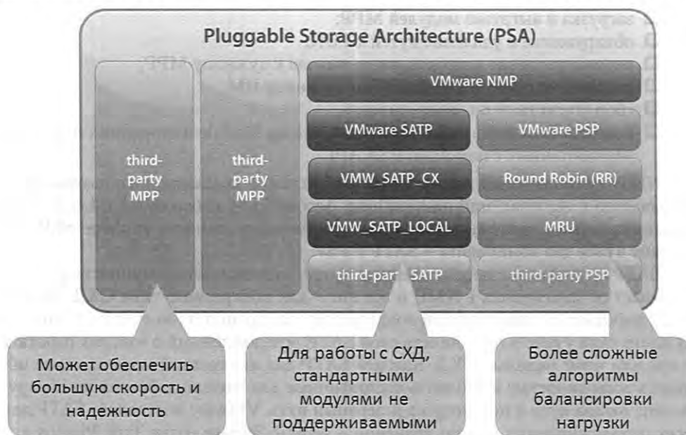
Рис. 3.11. Схема сосуществования встроенного и сторонних модулей multipathing Источник: VMware
