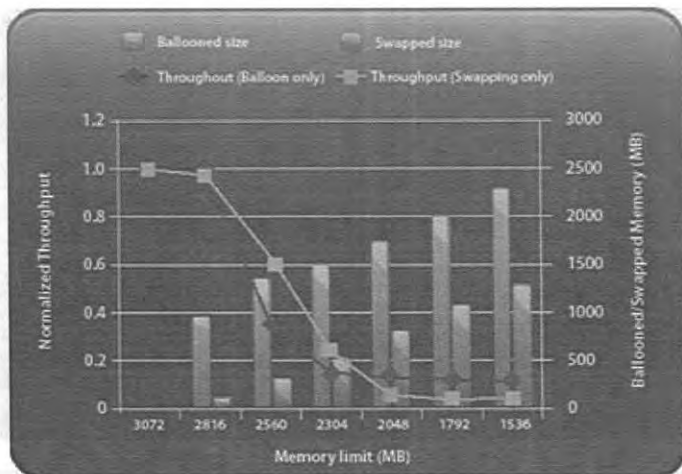
Рис. 6.36. Количество транзакций в секунду для SPECjbb при отъеме памяти с помощью balloon или vmkernel swap
