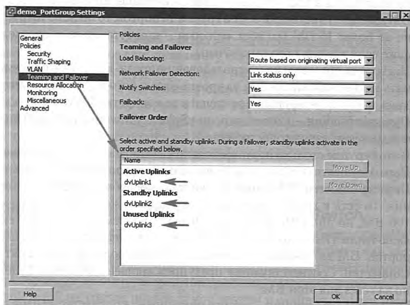
Рис. 2.17. Настройки использования внешних подключений для группы портов на dvSwitch
