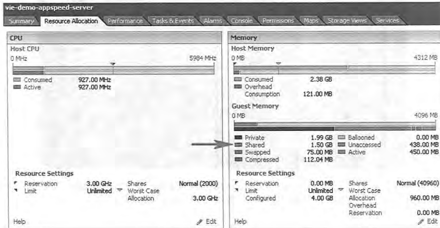
Рис. 6.29. Выделение памяти для одной ВМ
