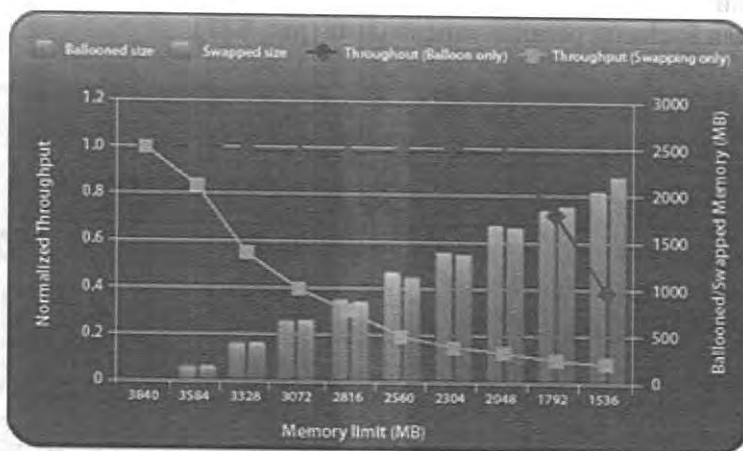
Рис. 6.35. Количество транзакций в секунду для БД Oracle при отъеме памяти с помощью balloon или vmkernel swap
