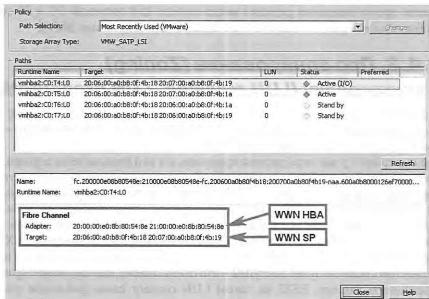
Рис. 3.14. Информация о путях к LUN
