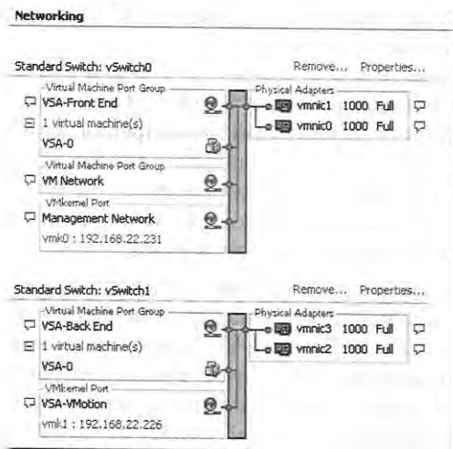
Рис. 3.44. Сетевые объекты, добавленные при настройке VSA
