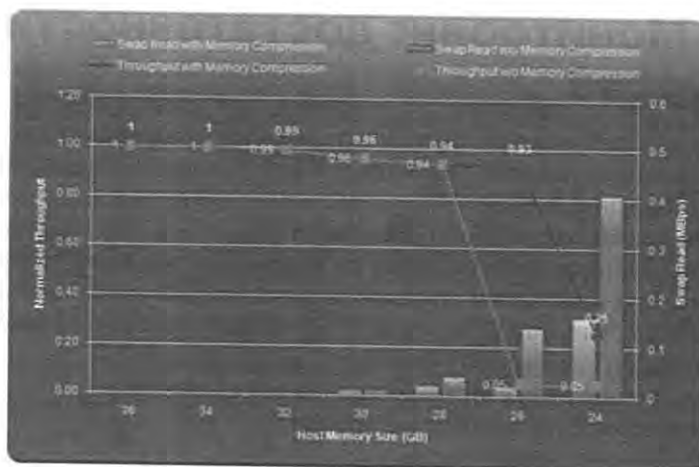
Рис. 6.38. Отъем памяти у сервера SharePoint механизмами memory compression и vmkernel swap
