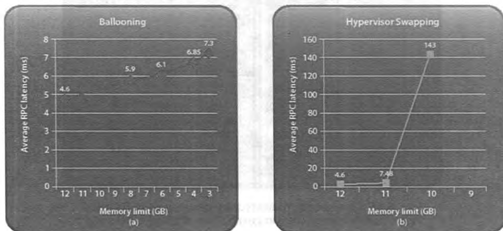
Рис. 6.37. Задержки при обработке почты сервером Exchange при отъеме памяти с помощью balloon или vmkernel swap
