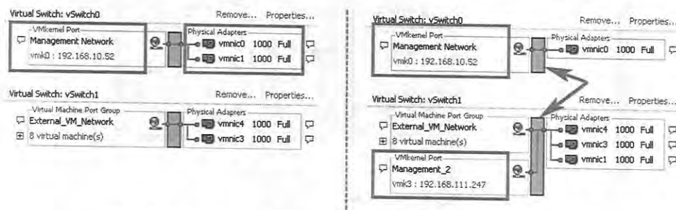
Рис. 7.9. Схемы дублирования управляющих интерфейсов
